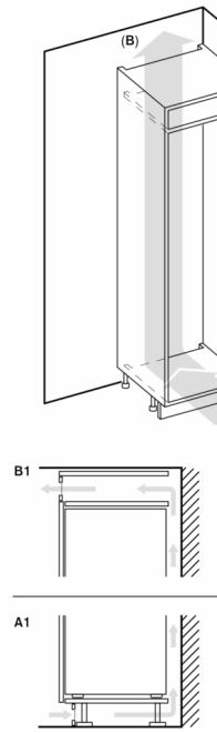
A: Lufteinlass \geq 200 \text{ cm}^2 ; Belüftungsr B: Luftauslass \geq 200 \text{ cm}^2 ; Belüftungsr
