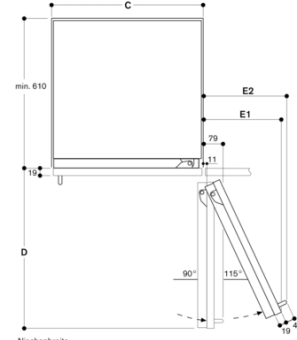
In der Zeichnung wurde eine Möbelfrontdicke von 19 mm sowie die Höhe eines Gaggenuu Möbelgriffs von 49 mm zugrunde gelegt.
