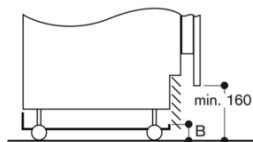
Seitenansicht Sockelbereich
