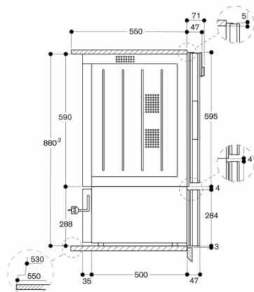
Seitenansicht WS 462 unter BO
