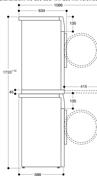
Seitenansicht WD 260 über WM 260 mit Verbindungssatz WA 032 001
