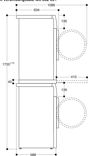
Seitenansicht WT 260 über WM 260 mit Verbindungssatz WA 032 001
