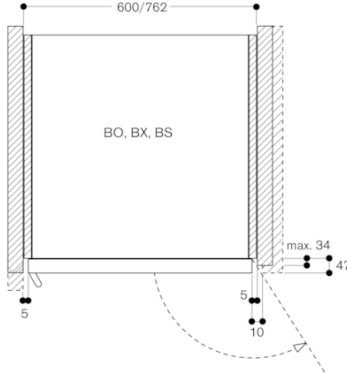
Luftquerschnitte an den Türkanten
