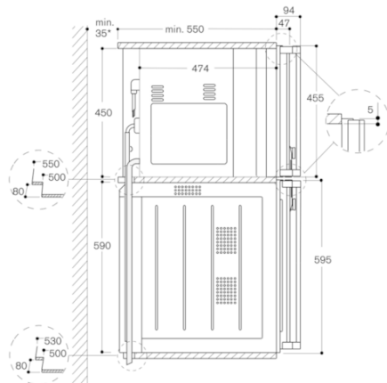
Einbau BS 270 über BO, Seitenansicht
