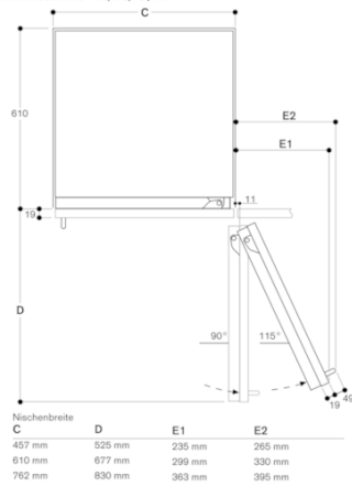
In der Zeichnung wurde eine Möbelfrontdicke von 19 mm sowie die Höhe eines Gaggenau Möbelgriffs von 49 mm zugrunde gelegt.
