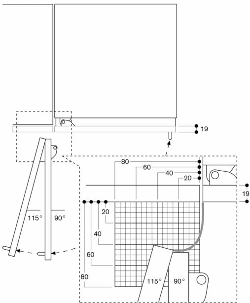
Türöffnungswinkel
