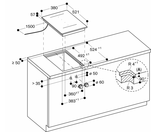
A: 6,5 +0,5 Maße in mm
