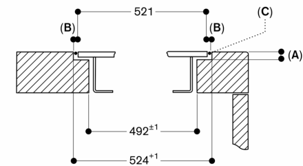
A: 6,5 +0,5 B: 1,5 C: Füllung mit Silikon Maße in mm
