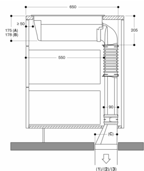
Abluftbetrieb mit Gebläsebauteil 1: AR 403 2: AR 400 3: AR 401 A: Aufgesetzter Einbau B: Flächenbündiger Einbau C: 152,5 Maße in mm
