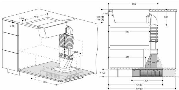
A: Aufbauanmontage B: Flächenbündiger Einbau (nur VL 414) C: Filterzugang von der Vorderseite D: Filterzugang von der Rückseite Anschlussstutzen flach/rund zur Vorderseite Anschlussstutzen flach/rund zur Rückseite Nicht empfohlen für nicht wärmeisolierte Böden ( U \geq 0,5 \text{ W/m}^2\text{K} ) Maße in mm
