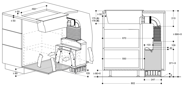
A: Aufbauanmontage B: Flächenbündiger Einbau (nur VL 414) Nicht empfohlen für nicht wärmeisolierte Böden ( U \geq 0,5 \text{ W/m}^2\text{K} ) Maße in mm
