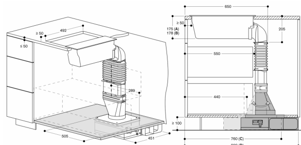
A: Aufgesetzter Einbau B: Flächenbündiger Einbau (nur VL414) C: Abluft nach links, flacher/runder Anschlussstutzen zur Front D: Abluft nach rechts, flacher/runder Anschlussstutzen zur Rückseite Maße in mm
