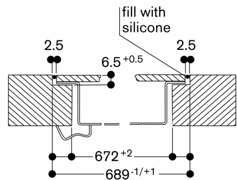
Longitudinal section
