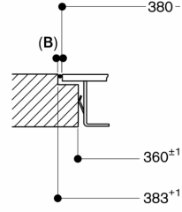
Longitudinal section
