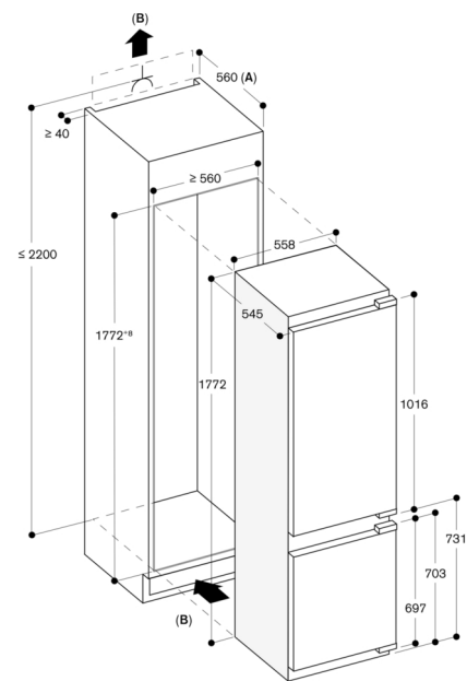
A: 560 mm recommended, min. 550 mm B: min. 200 cm 2 A: Socket
