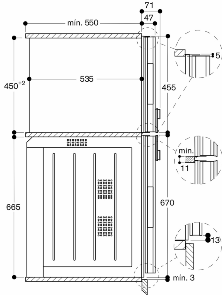
Vista lateral BM 484/485 sobre BO
