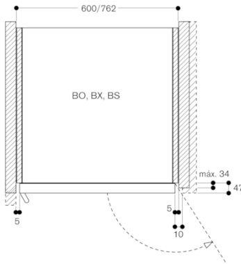
Secciones transversales de aire en los cantos de la puerta
