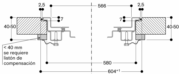
Sección transversal
