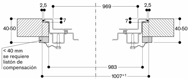
Sección longitudinal
