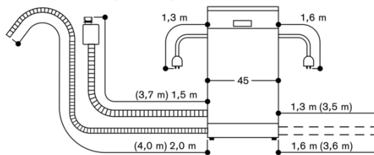
Medidas de conexión para lavavajillas de 45 cm ancho
