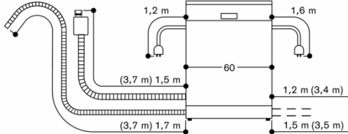
Medidas de conexión para lavavajillas de 60 cm ancho
