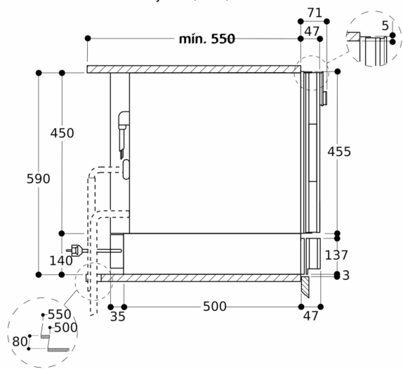
Vista lateral DV 461 bajo BS, BM, CM
