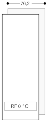
Distancia a la pared RB 472/RC/RF/RW
