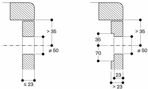
Montaje de los mandos reguladores, montaje superpuesto
