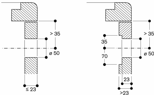
Montaje de los mandos reguladores, montaje enrasado
