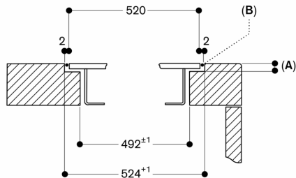
Sección transversal
