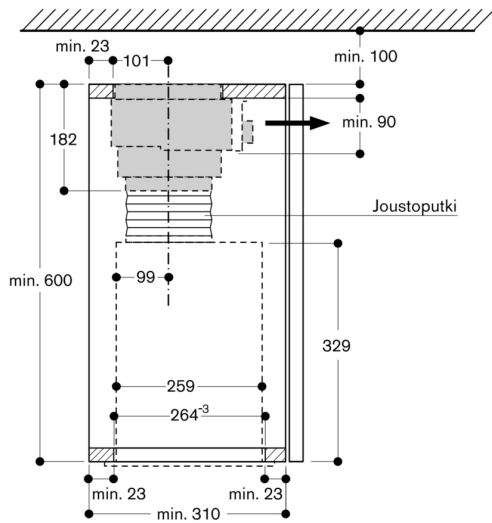
Poikkileikkaus yläkaapista kun AC 200 ja AA 211 812
