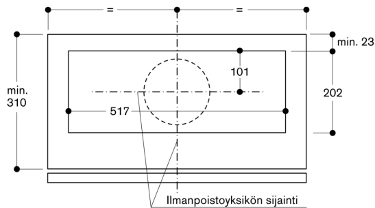
Kuva yläkaapista ylhäältä kun AC 200 ja AA 211 812
