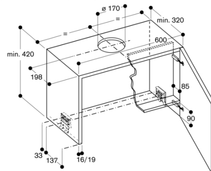
Yläkaappi mallille AF 200 160
