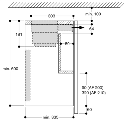
Poikkileikkaus yläkaapista kun AA 211 812 ja laskeutuva kehys AA 210 490/460
