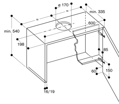
Yläkaappi mallille AF 200 160 kun laskurunko AA 210 460
