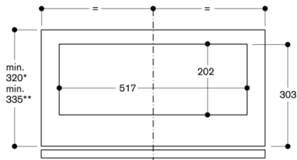
Kuva yläkaapista ylhäältä kun AA 211 812
