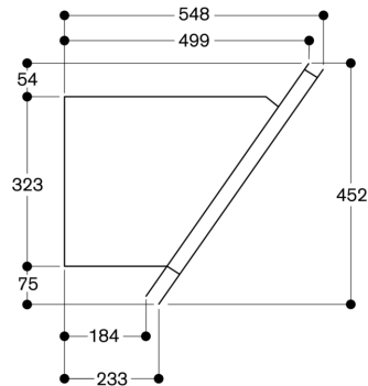
Sivukuva
