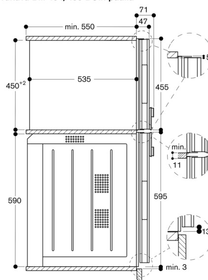
Sivukuva BM 454/455 BO:n päällä
