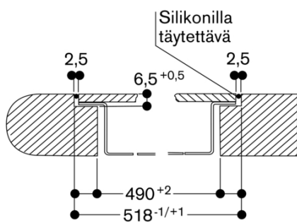
Poikkileikkaus
