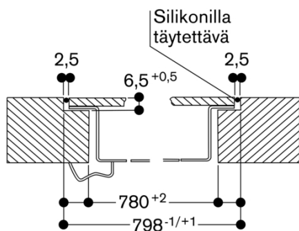
Pitkittäisleikkaus
