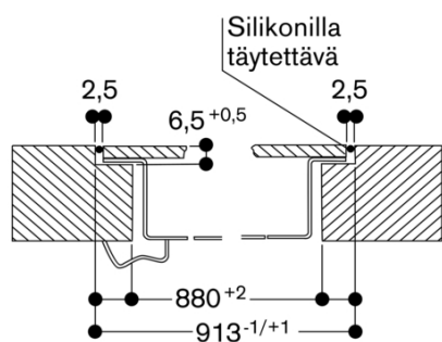
Pitkittäisleikkaus
