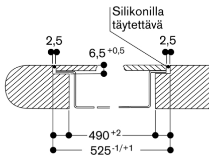
Poikkileikkaus
