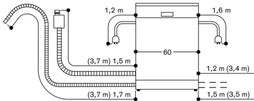
Liitäntämitat 60 cm leveälle astianpesukoneelle
