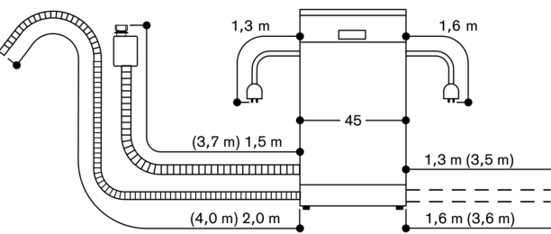
Liitäntämitat 45 cm leveälle astianpesukoneelle
