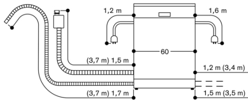
Liitäntämitat 60 cm leveälle astianpesukoneelle
