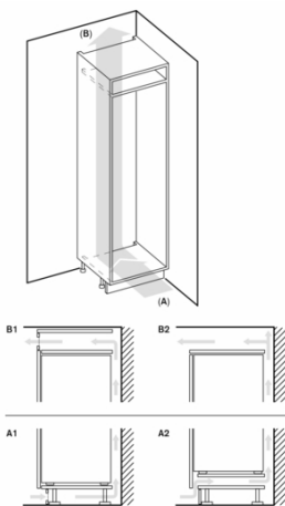
A: Ilmantuloaukko \geq 200 \text{ cm}^2 ; ilmankiertovalttoehdot A1 tai A2 B: Ilmanlähtöaukko \geq 200 \text{ cm}^2 ; ilmankiertovalttoehdot B1 tai B2
