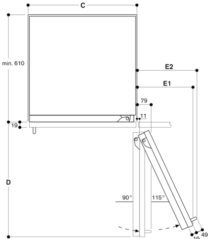
Asennussyvennyksen leveys
