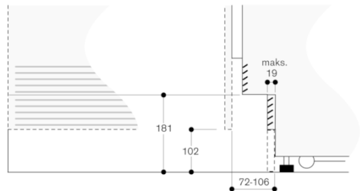
Kun kyseessä laitteen vakiokorkeus ja sokkelilistan korkeus 102 mm. Sokkelilistan maksimivahvuus 19 mm.
