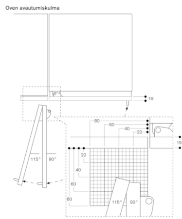
Saranan avautumiskulma ja siitä seuraavat, paneelin paksuudesta riippuvat etäisyydet viereisiin kalusteisiin ja ovenkahvoihin ilmenevät oikeasta piirroksesta. Piirroksessa on oletuksena kalusteen paneelin paksuus 19 mm.
