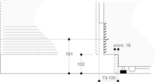
Yksityiskohta sokkelista
