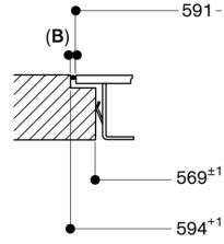
Pitkittäisleikkaus
