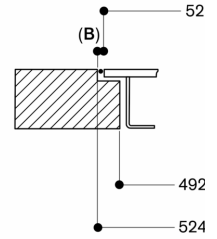
Poikkileikkaus
