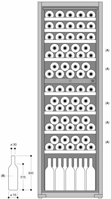
A: Zone adaptée au stockage de bouteilles magnum dans une configuration de plateau standard B: 0,75 litres Mesures en mm
