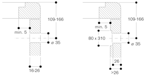
Installation du bouton de commande, encastrément affleurant
