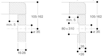
Installation du bouton de commande, montage sur le plan de travail
