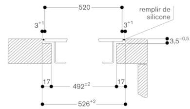
Coupe transversale
