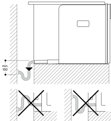
Raccordement d'eaux usées
