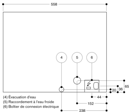
Vue de derrière
