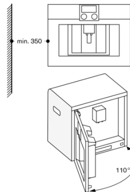
Montage en angle côté gauche
