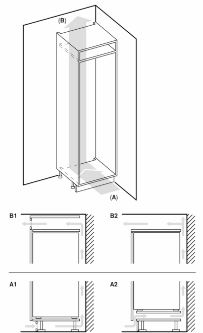
A: Entrée d'air \geq 200 \text{ cm}^2 ; options d'apport d'air supplémentaire A1 ou A2 B: Sortie d'air \geq 200 \text{ cm}^2 ; options de ventilation B1 ou B2
