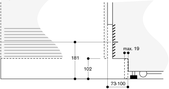
Détail plinthe
