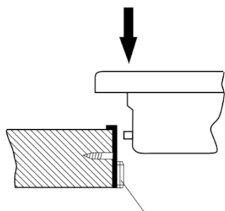
Rail de montage (arrière et avant)
