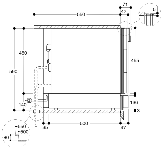
Vue de côté WS 461 sous BS, BM, CM
