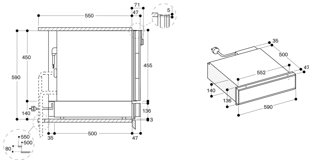
Vue de côté WS 461 sous BS, BM, CM
