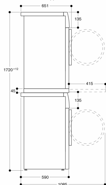
Vue latérale de WT 260 au-dessus de WM 260 avec kit de raccordement supplémentaire
