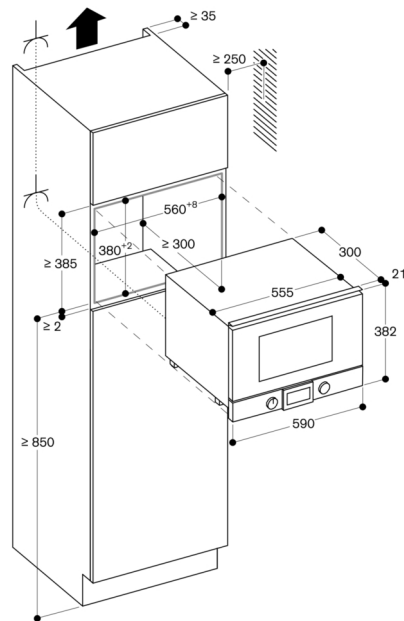
Installation dans un meuble haut
