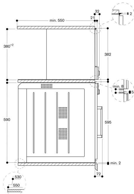
Vue latérale du BMP 224/225 au-dessus du BOP
