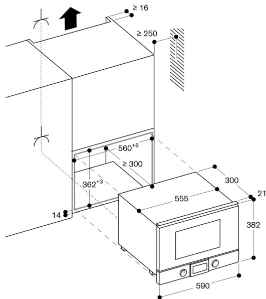
Montage dans élément haut
