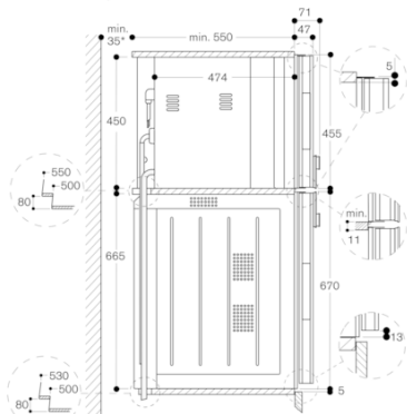
Vue latérale BS 484/485 au-dessus de BO
