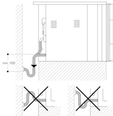
Raccord d'évacuation d'eau
