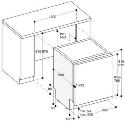
Lave-vaisselle plus haut de 81,5 cm avec charnière flexible
