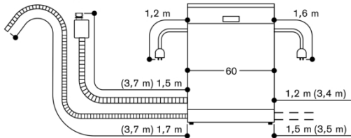
Dimensions de raccordement pour un lave-vaisselle de 60 cm de large
