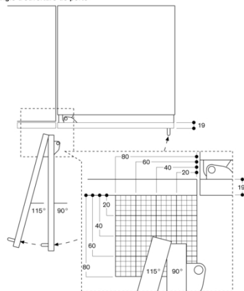
Angle d'ouverture de porte
