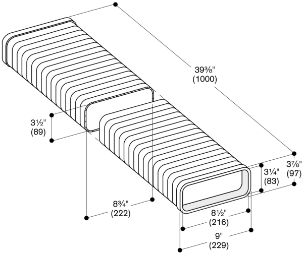
Dimensioni in pollici (mm)
